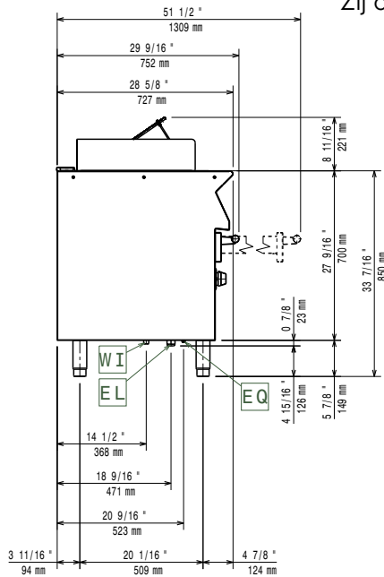
Zij aanzicht
